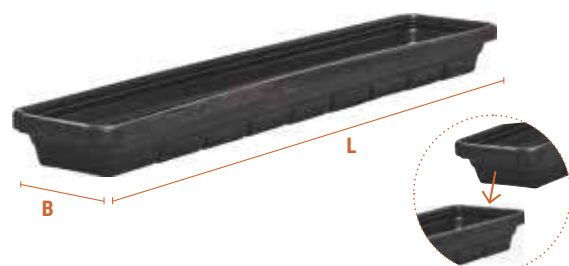
POB 150.057 L: 1,50 m - B: 0,57 m 7,0 kg POB 250.047 L: 2,50 m - B: 0,47 m 12,2 kg POB 300.047 L: 3,00 m - B: 0,47 m 12,4 kg
