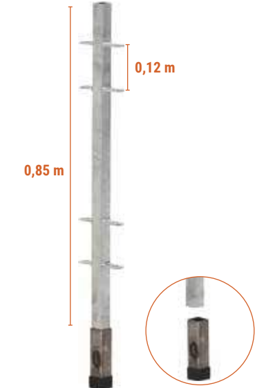
SPI 085DL2 2,9 kg
