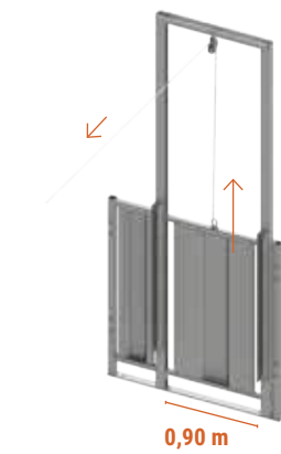
ILOP 90MT 36,4 kg
