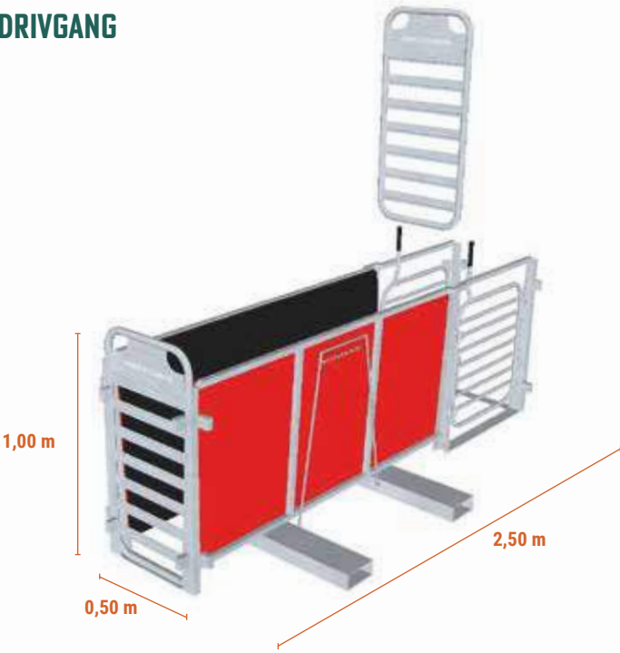
LQ VENO-F L: 2,50 m - H: 1,00 m - B: 0,50 m 180,0 kg
