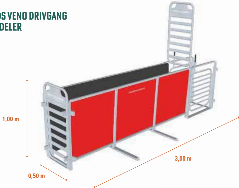
LQ VENO-T L: 3,00 m - H: 1,00 m - B: 0,50 m 140,0 kg
