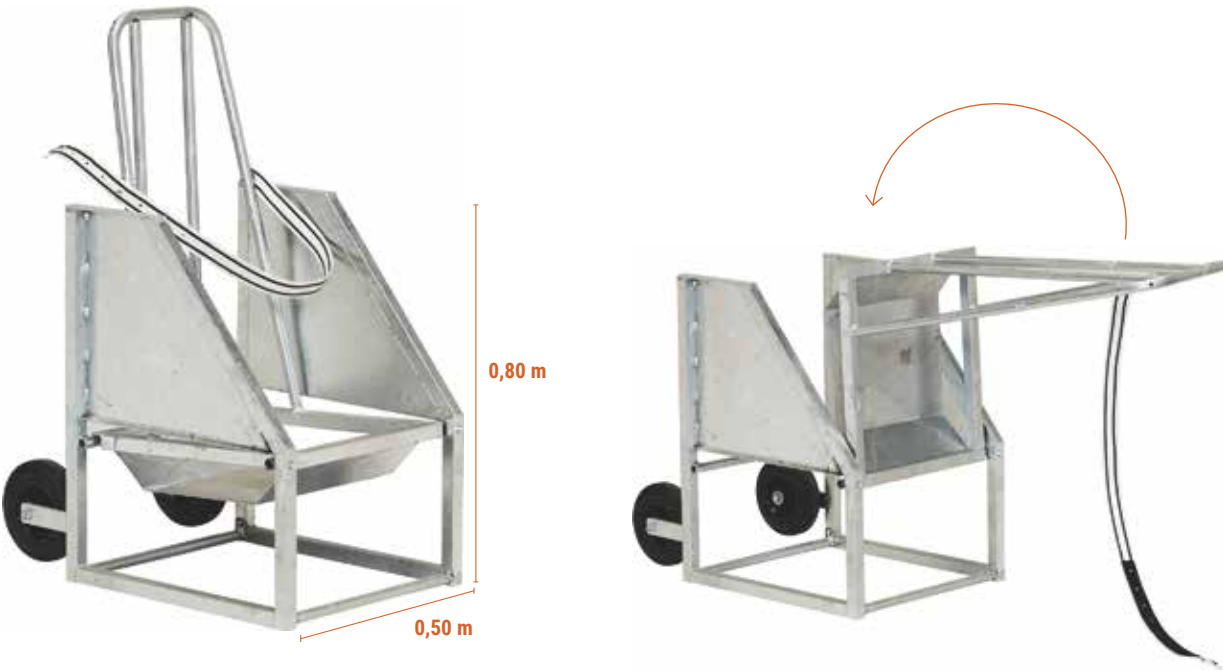
SS 050.080 B: 0,50 m - H: 0,80 m 24,5 kg
